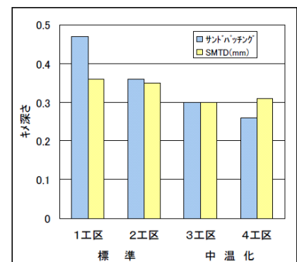
図-2 各工区のキメ深さ
