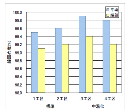
図-1 各工区の締固め度
