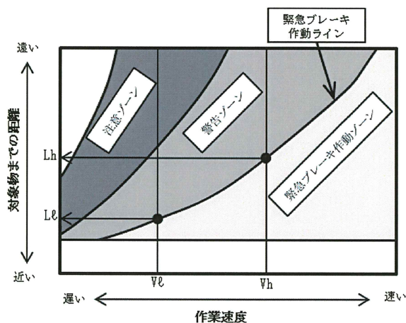
図-4 緊急ブレーキタイミング
