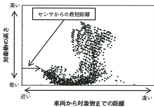
図-2 3Dセンサの検知データの例
